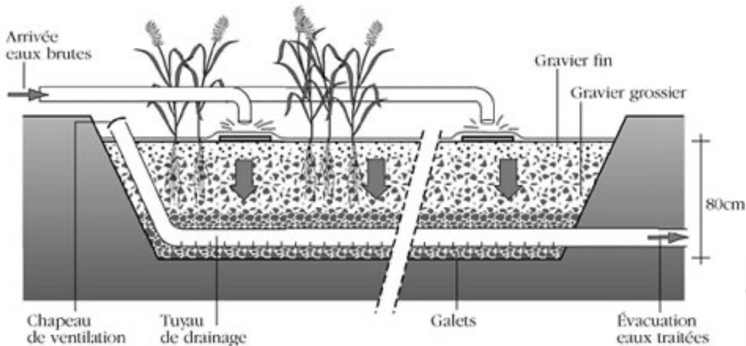
Schéma d'un filtre à écoulement vertical
